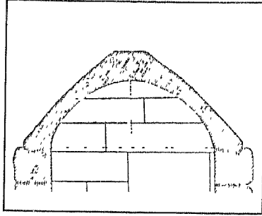
شكل (١٣) عقد قطع في سقف منح عرضه ٢ م . في الهرم الشمالي المنى باللى ندهسور الاسره النايه عسره .
